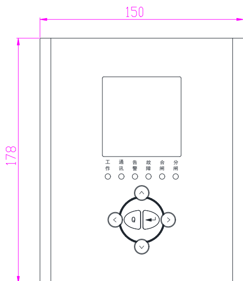
图 8.1 装置正视图
