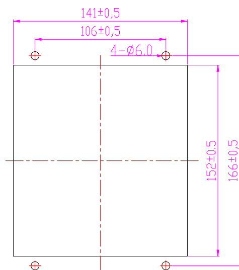
图 8.4 装置安装开孔图
