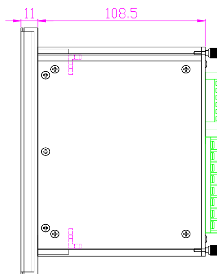
图 8.2 装置侧视图
